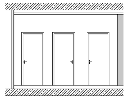
Wandansicht 8
