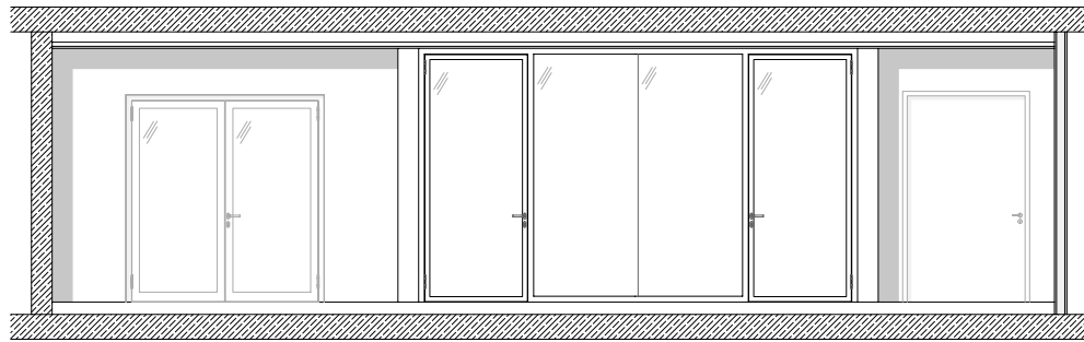
Wandansicht 3 Stütze Sichtbeton Stütze Sichtbeton
