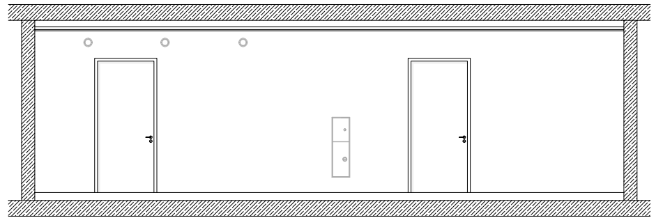
Wandansicht 4 Entnahmekasten Trockensteigleitung Schutzschrank Feuerlöcher
