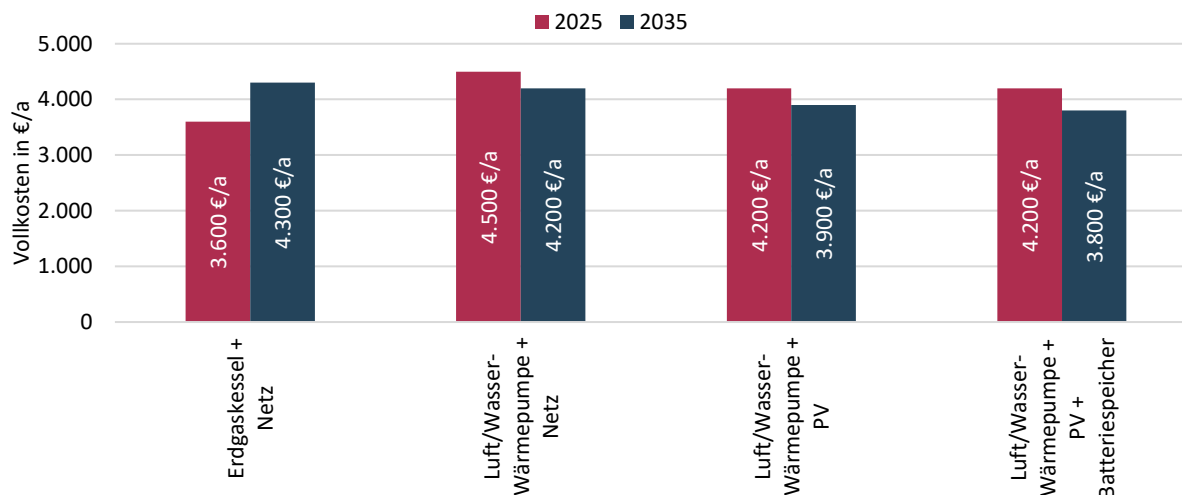
Abbildung 45: Typische Vollkosten der Energieversorgung für ein Einfamilienhaus
