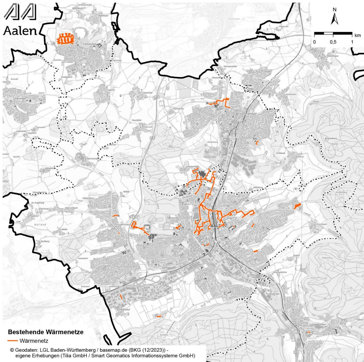
Abbildung 10: Trassenverlauf bestehender Fernwärmenetz Aalen
