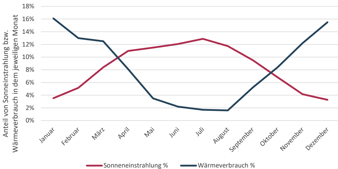
Abbildung 21: Saisonale Verteilung der Sonneneinstrahlung und des Wärmeverbrauchs in Aalen
