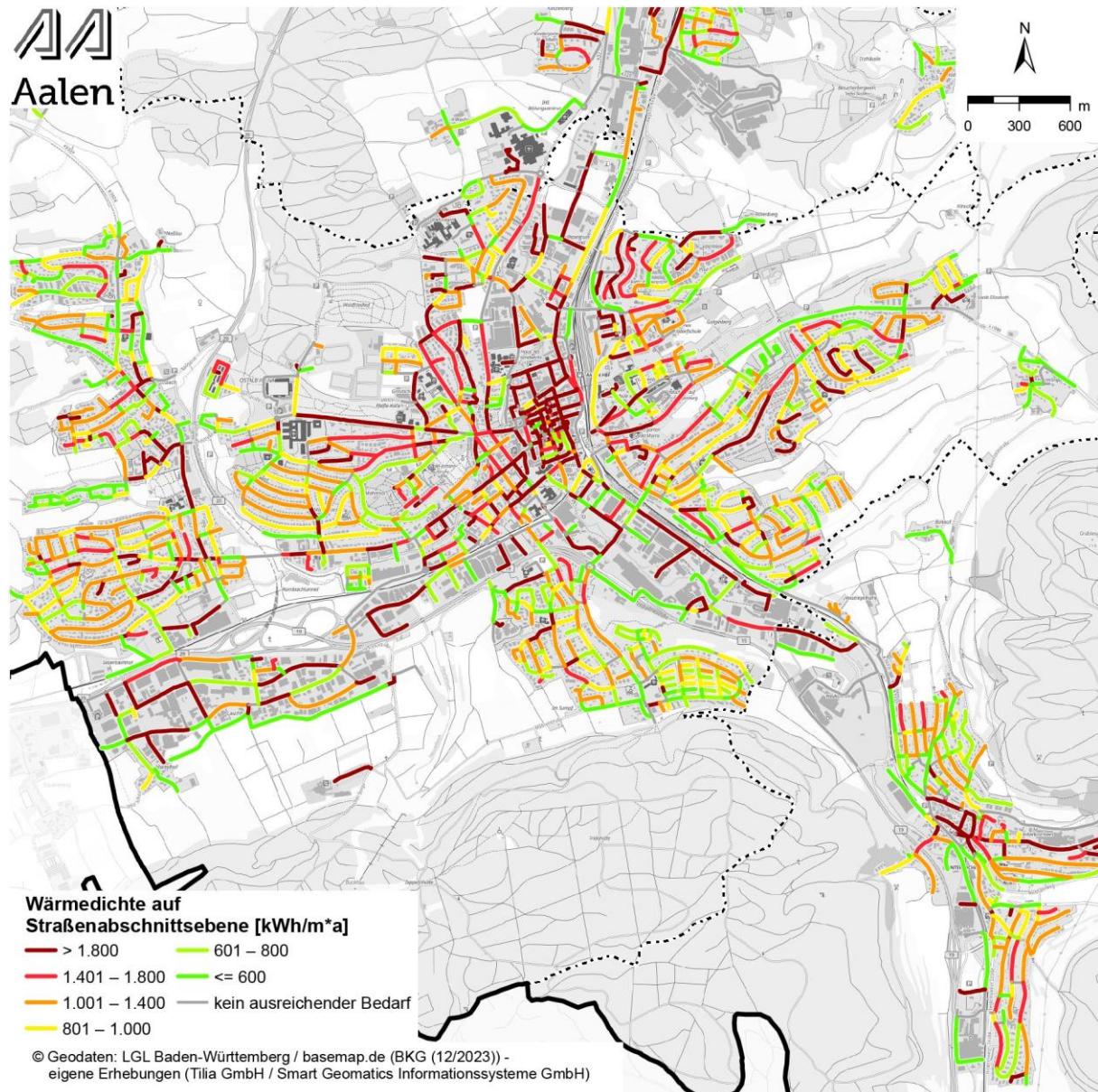
Abbildung 7: Übersicht Wärmelinienichten (ohne HAL) im Stadtgebiet Aalen
