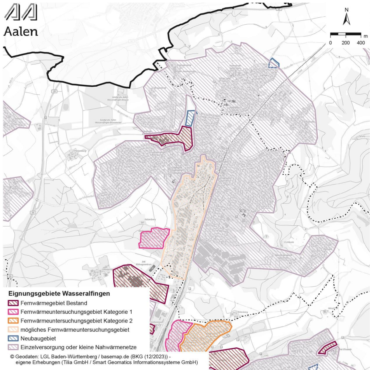
Abbildung 38: Übersicht der Eignungsgebiete nach Kategorien in Aalen – Wasseralfingen - Hofen
